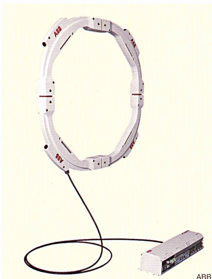
Bild 2 Faseroptischer Stromsensor mit Steuer- und Regelsystem
