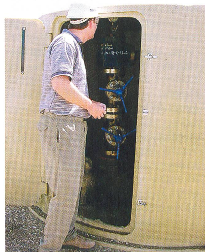
Injecteur CO 2 .
