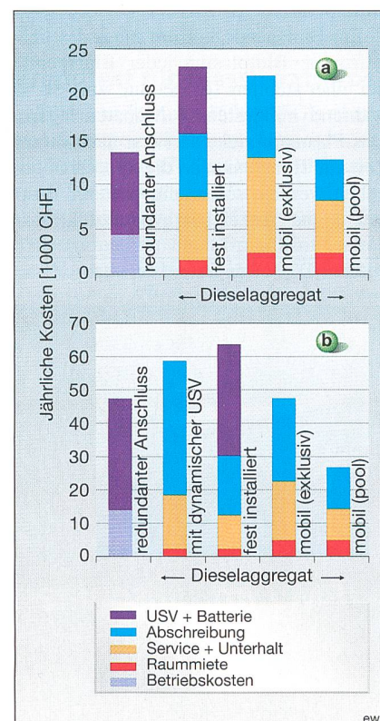
Bild 5 Jährliche Kosten verschiedener Notstromanlagentypen
