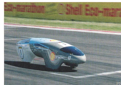
Der PAC-Car II während dem Shell-Eco-Marathon in Nogaro: Mit dem Äquivalent von einem Liter Benzin hat das Brennstoffzellen-Fahrzeug auf seiner Rekordfahrt 5134 Kilometer zurückgelegt.
