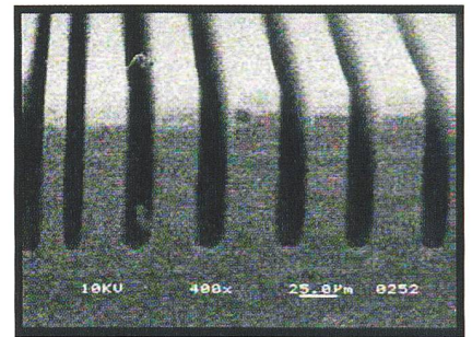
Brennstoffzelle: Elektroden-Mikrostruktur (Bild PSI).
