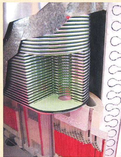
Brennstoffzellenstapel.
