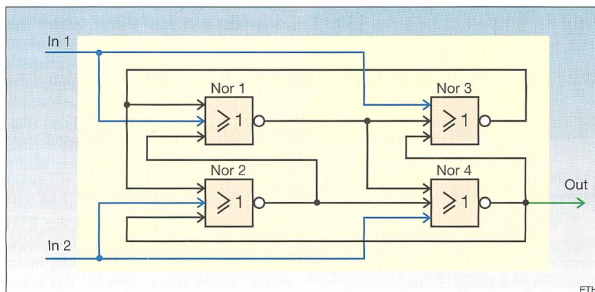
Bild 5b Speichereinheit aus 4 Nor-Gattern
