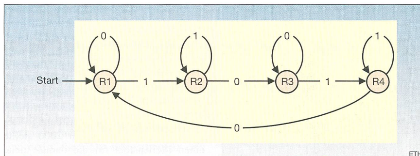
Bild 5a Funktionsweise der Speichereinheit (Zustandsautomat)
