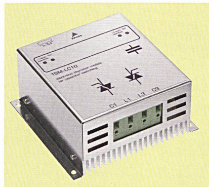
Kompaktes Thyristormodul zur Blindleistungskompensation
