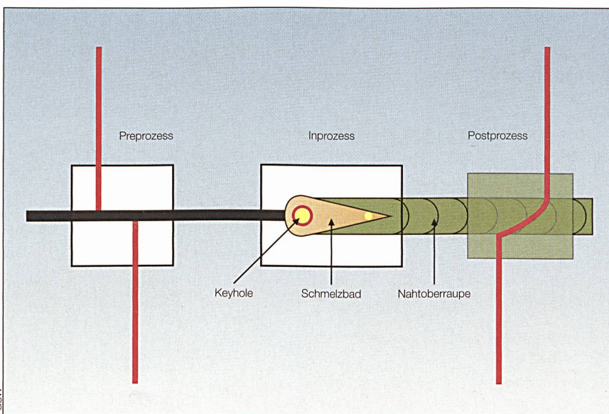
Bild 5 Laserschweißen überwachen.
