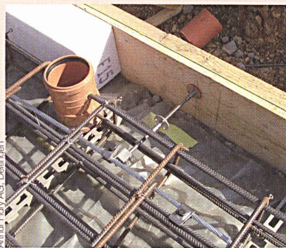
Erdenseil (Stahl 75 mm 2 ) mit Fundamenterdungsanschlussgarnitur und korrosionsfester Verlängerung für die Isolation.
