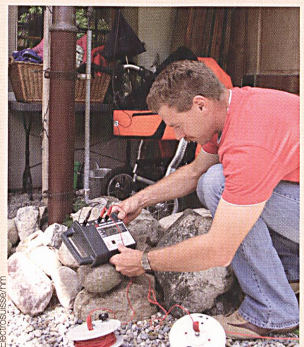
Widerstandskontrolle einer bestehenden Erdung an einem ehemaligen Landwirtschaftsgebäude. Das Messergebnis von 12 Ω ist für eine bestehende Anlage in Ordnung; neue Tiefenerdungen nach SEV 4022:2004 sollten ein Ergebnis unter 10 Ω erreichen. Das Gebäude ist zwar nicht blitzschutzpflichtig; weil aber eine Blitzschutzanlage aus dem Jahre 1984 vorhanden ist und das Gebäude saniert wird, verbunden mit einer grösseren Wertvermehrung, muss die Anlage entweder der Norm SEV 4022:2004 entsprechen, oder sie muss entfernt werden.
