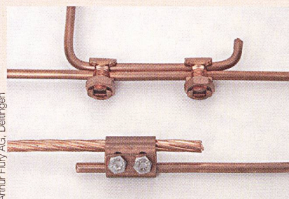
Oben: Erdseil 50 mm 2 auf Kupferdraht mit korrodiertem Kreuzverbinder. Unten: Korrekte Verbindungen im Erdreich.
