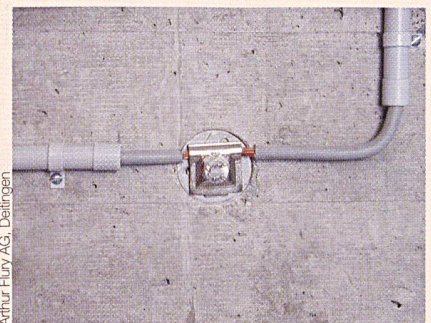
Fundamenterdungs-Anschliesspunkt, korrosionsfest (Inox A4), mit Potenzialausgleichsleitung.
