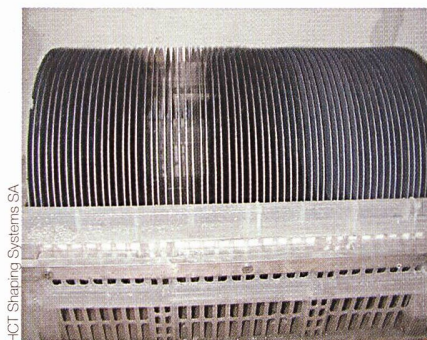
Drahtschneidemaschine von HCT Shaping Systems SA.
