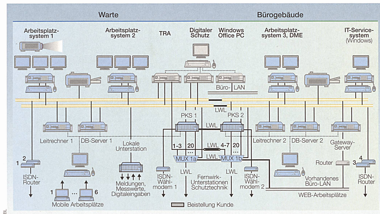
Bild 2 Aufbau des Netzeitsystems bei EBL.
