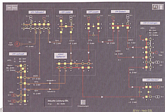
Bild 3 Bildschirmabbildung des 50-kV-Netzes.
