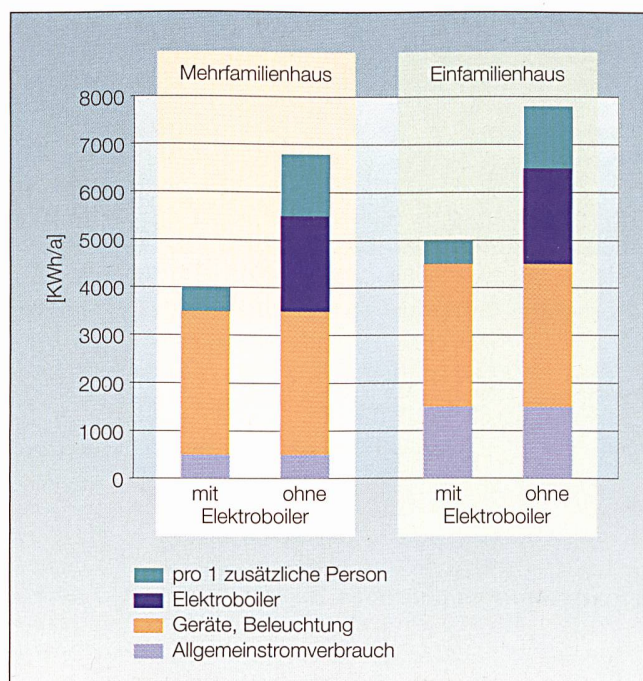
Bild 1 Typischer Haushalt-Stromverbrauch.
