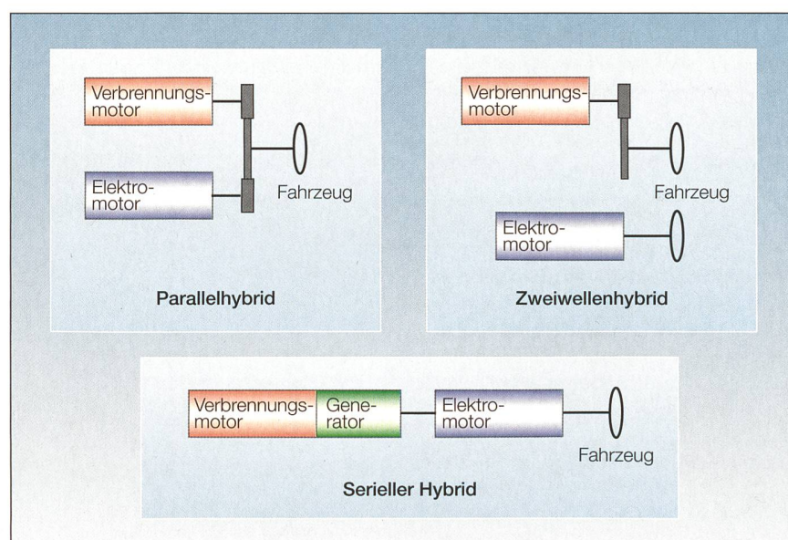
Bild 1 Struktur von Hybridantrieben.
