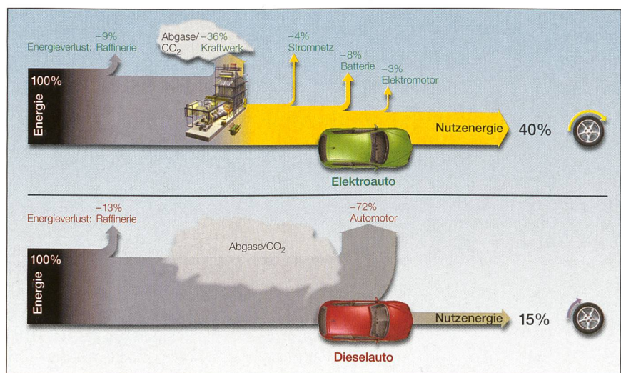
Bild 1 Effizienzvorteile des Elektroantriebs: Energiekette. Vergleich der Energieeffizienz (Well-to-Wheel) Dieselauto/Elektroauto.
