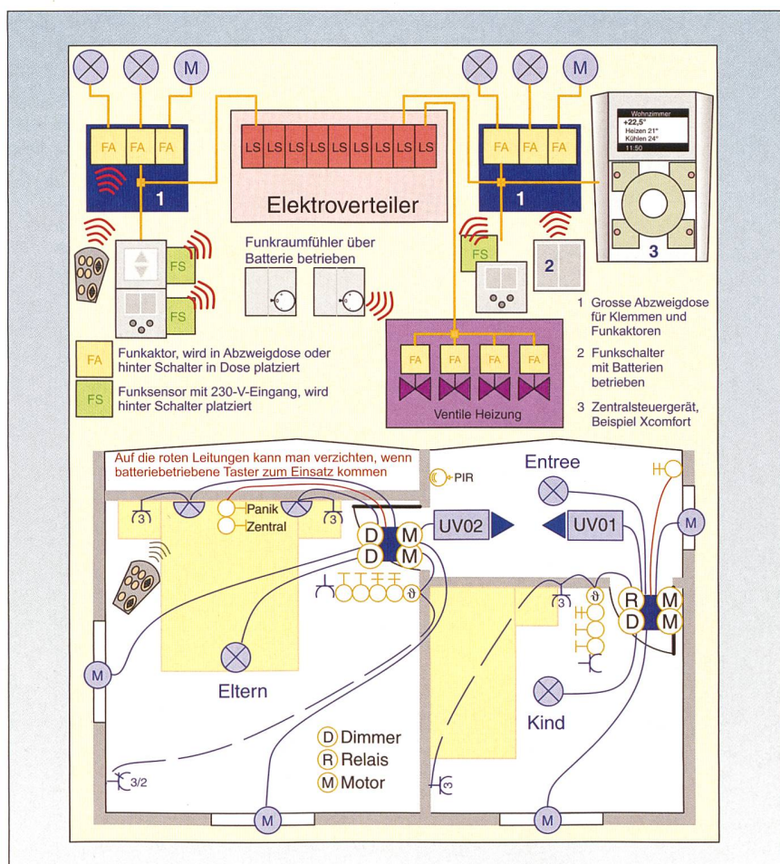
Bild 7 Prinzip eines funkbasierenden Systems.
