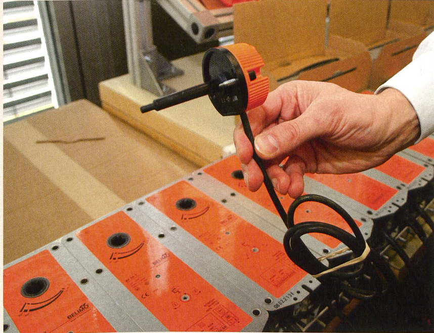
Die fertigen Brandschutzklappenantriebe mit den Thermoelementen aus der Sonnhalde – bereit für die Auslieferung nach ganz Europa.
