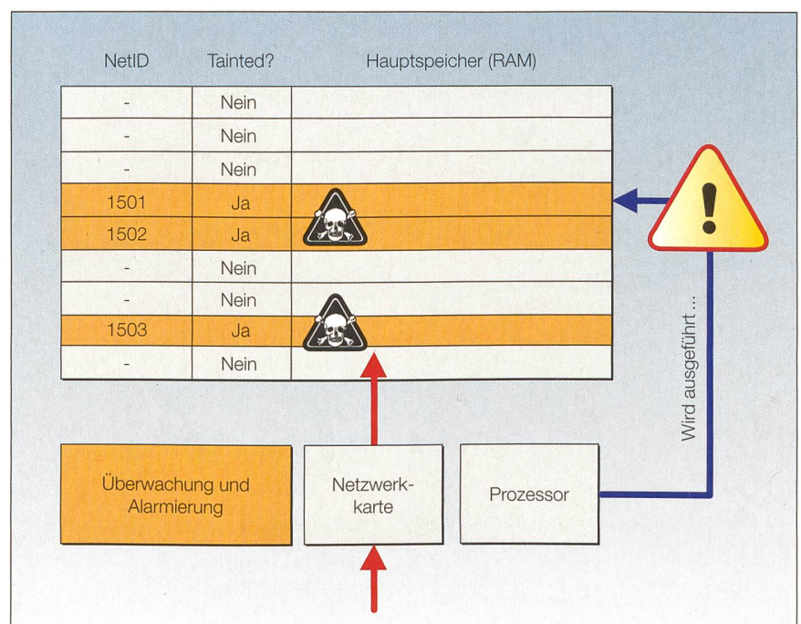
Bild 5 Markieren von potenziell gefährlichen Daten (Memory Tainting).
