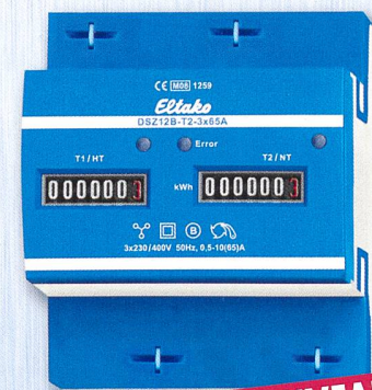
E-No 981 873 118 max. 3x65 A, 3x230/400 V avec double tarif Capot plombable
