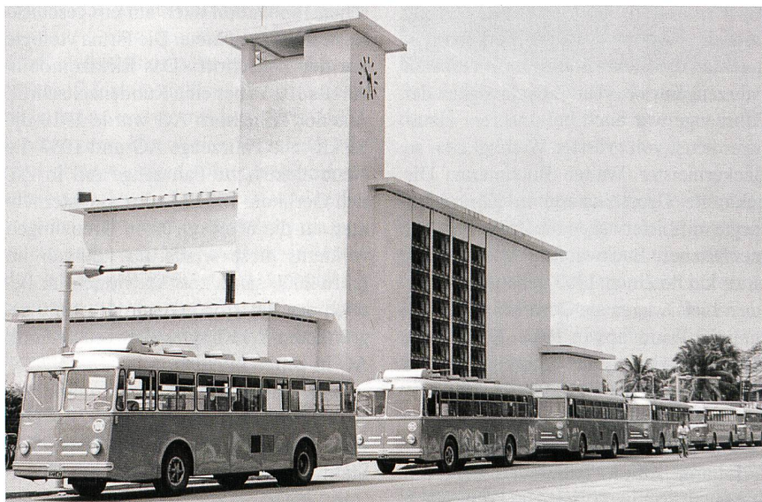
Für Léopoldville (heute Kinshasa) baute MFO 12 Gyrobusse, welche ab 1955 auf zwei Linien verkehrten.
