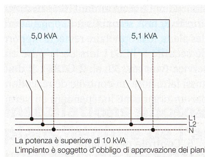
Figura 2 Impianti polifase.
