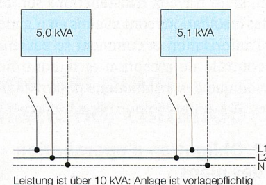
Bild 2 Mehrphasige Anlagen.
