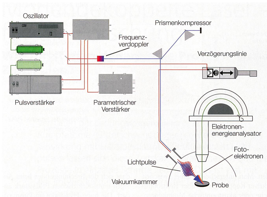
Bild 4 Typischer Aufbau eines zeitaufgelösten Fotoemissionsexperiments: Lichtpulse aus einem Oszillator (Verstärker, halb transparent dargestellt) werden in zwei Pulse geteilt (Pumpimpuls und Abfrageimpuls). Je nach Bedarf kann die Frequenz der Pulse z.B. in doppelbrechenden Kristallen vervielfacht werden.
