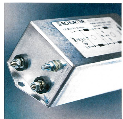
Schurter-Netzfilter speziell für Frequenzumformer, Schrittmotor-Antriebe, USV-Anlagen usw.
