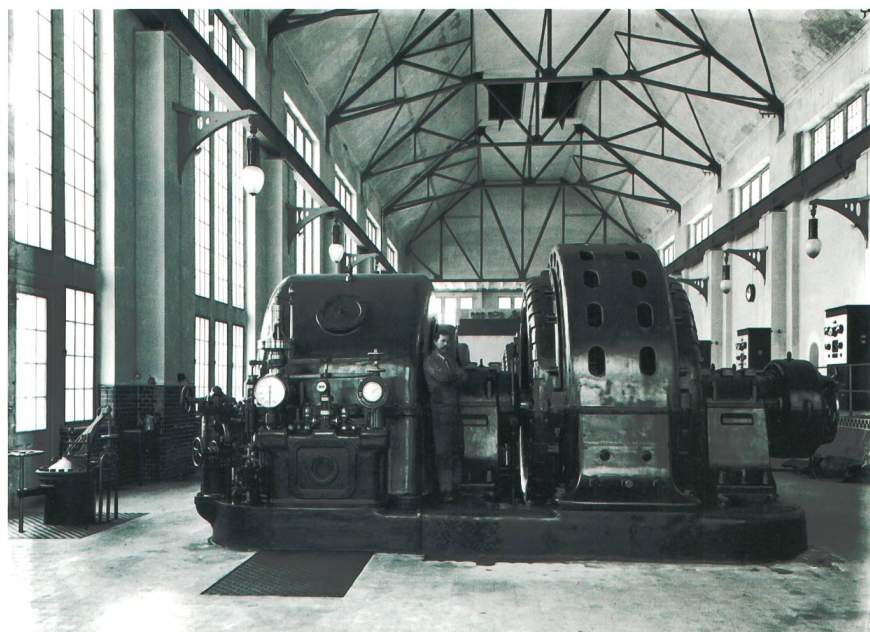
Mit der Eröffnung des Löntschwerks 1908 erhielten die Elektrizitätswerke im Glarner Mittel- und Unterland einen zuverlässigen Lieferanten von Elektrizität.
