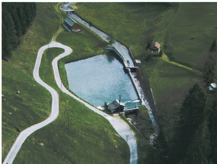
Das Kraftwerk am Niederenbach in Schwanden ist das älteste noch in Betrieb stehende Kraftwerk der kommunalen Elektrizitätswerke. Es wurde am 4. November 1899 mit einer maximalen Leistung von 760 PS eröffnet, mehrmals erweitert und weist heute eine maximale Leistung von 1760 kW auf.
