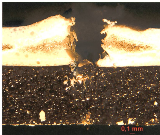
Die Membrane aus Polyvinylchlorid-Polyester wurde mit einer Nadel von 2,5 mm Durchmesser durchstoßen, worauf sich der Polyurethan-Schaum (braun) schlagartig ausdehnte.
