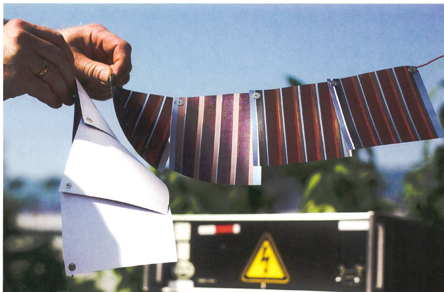
Die auf Papier gedruckten Solarmodule mit einem Wirkungsgrad von 1,3 % werden mit Druckknöpfen elektrisch verbunden und bilden eine Serienschaltung. Nach Gebrauch wandern sie ins Altpapier.
