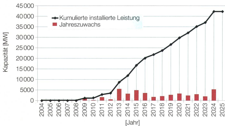
Bild 5 Geplanter Kapazitätzuwachs Offshore-Windkraft.
