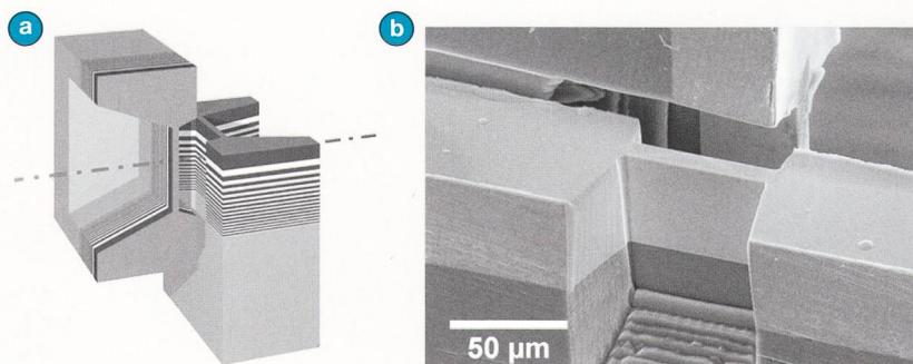
a) Schematische Darstellung zweier gekreuzter Multischicht-Laue-Linsen, b) REM-Aufnahme zweier gekreuzter MLL nach der FIB-Bearbeitung (in Zusammenarbeit mit Fraunhofer IKTS-MD).
