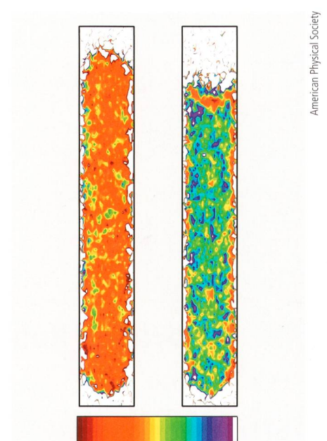
Räumliche Verteilung von Eis und Wasser in einer zylindrischen Wassersäule, wie sie in der vorliegenden Studie mit der neuen Neutronenbildgebungstechnik gemessen wurde. Rot: nur Eis vorhanden.
