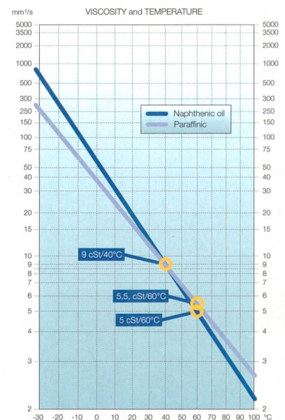
Viskositätsindex.
