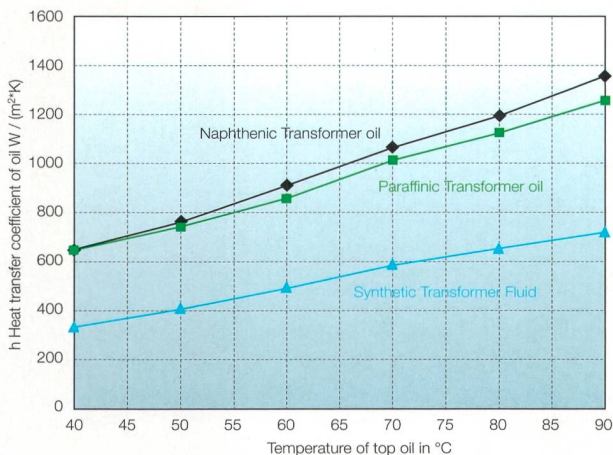
Wärmeübertragungskoeffizient.
