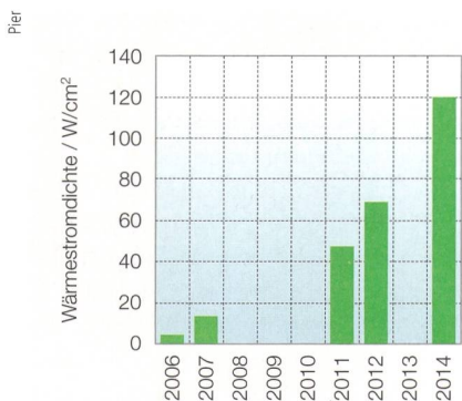
Bild 2 Entwicklung der Wärmestromdichte.
