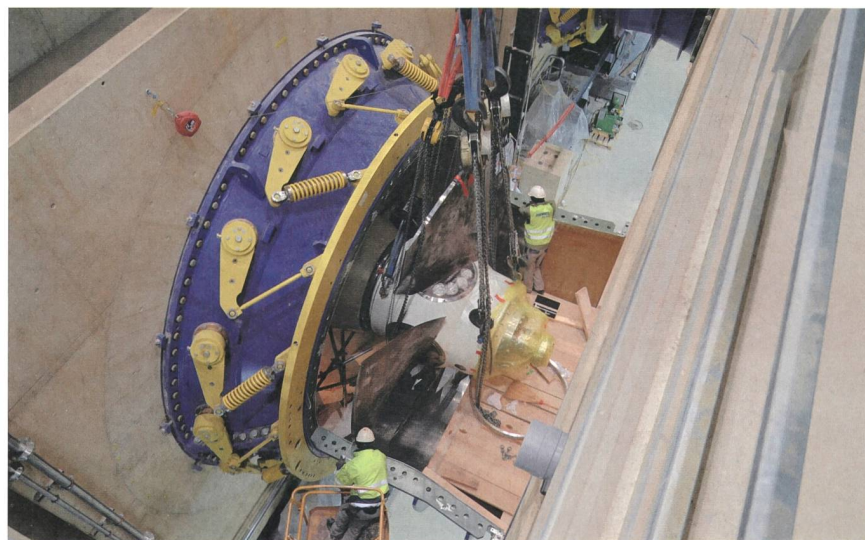
Figure 3 Mise en place d'une turbine bulbe Kaplan à axe horizontal.
