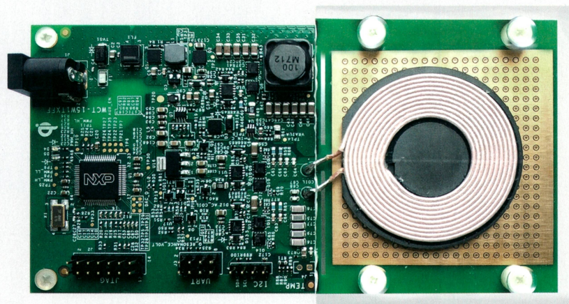
Referenz-Design eines einspuligen drahtlosen 15-W-Ladegeräts mit fester Frequenz von NXP Semiconductors.
