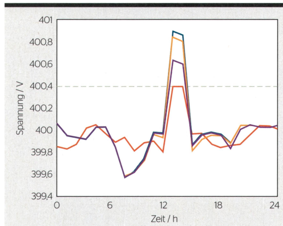
Bild 6 Spannungsvergleich:
