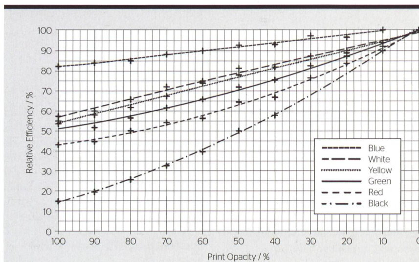
Bild 3 Zusammenhang zwischen der Deckkraft (Print Opacity) einer Grundfarbe und der resultierenden RE (Relative Efficiency) [2].
