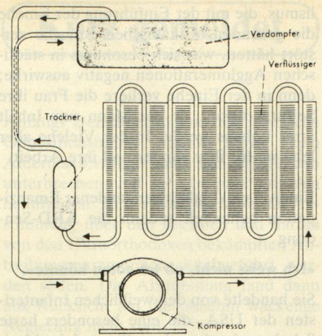
Kältemaschine: Funktionsschema
