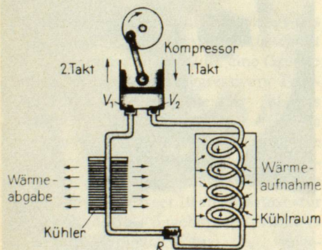
Kompressor-Kältemaschine: Schema
