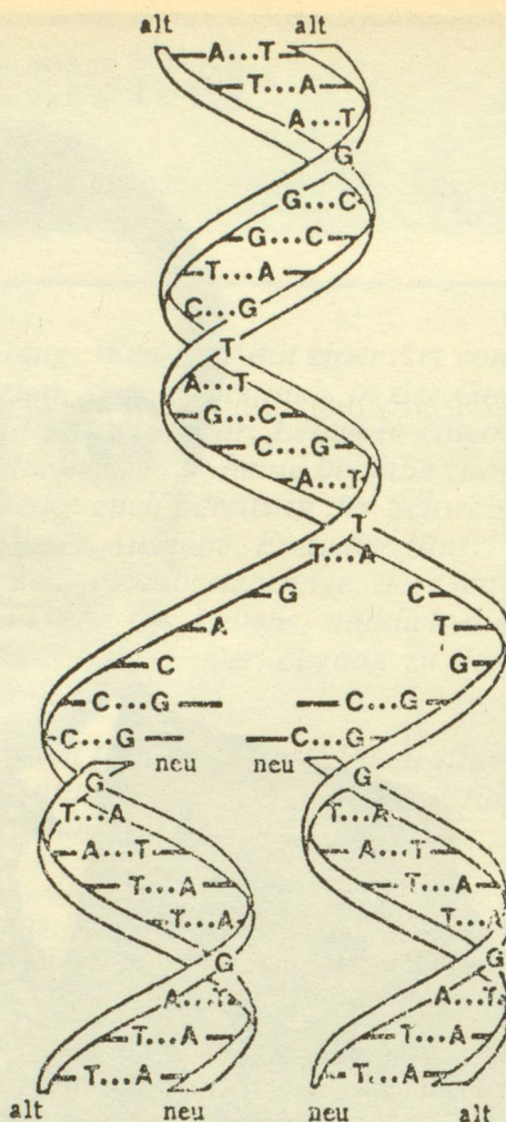
Schematische Darstellung des als Doppelstrang aufgebauten DNA-Moleküls im Begriff der Replikation. Diese Nukleinsäure, in den Chromosomen aller Zellen enthalten, ist Träger der genetischen Information.
