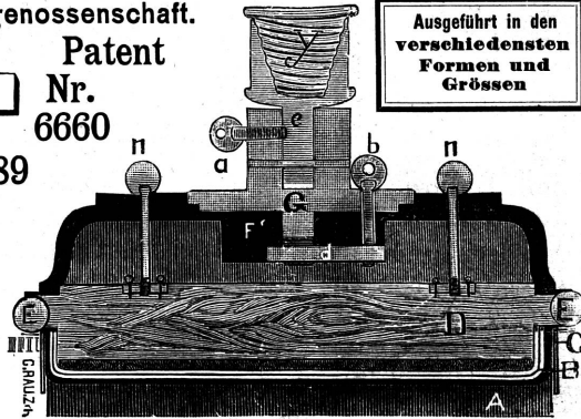
Durchschnitt einer Patent-Blochbürste.
