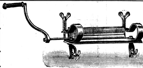
Patent-Waschmaschine mit Hebelbetrieb.
