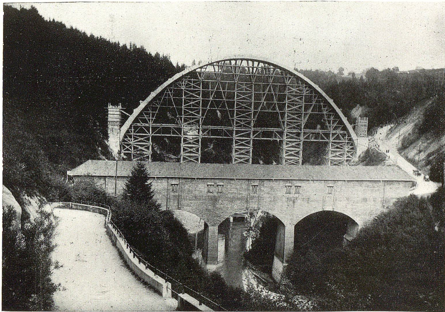
Die alte Brücke und das Leegerüst der neuen Brücke über die Urnäsch bei Hundwil. Phot. Willi Hofer.
