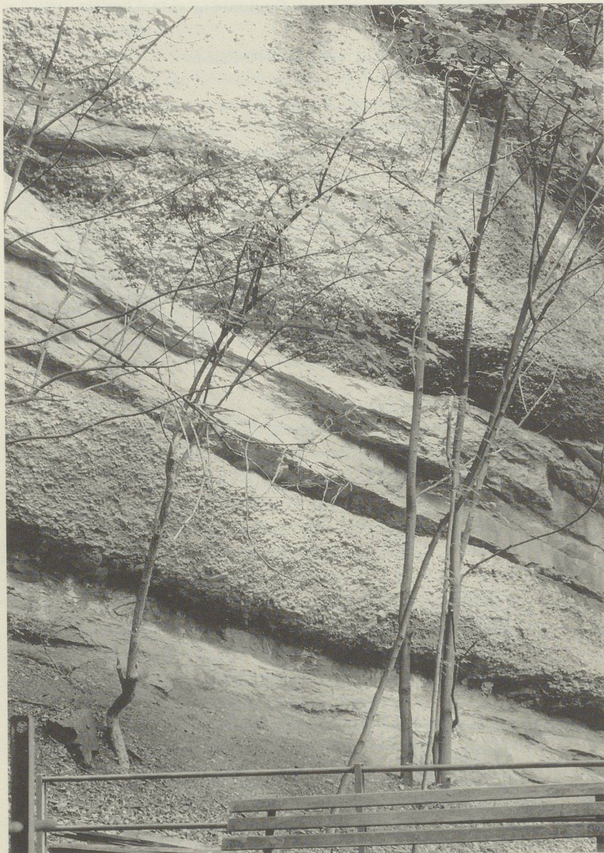
Knapp ausserhalb der St. Galler Altstadt öffnet sich in der Mühlenenschlucht ein geologisches Bilderbuch. Sandstein- und Mergelschichten wechseln mit Nagelfluhbänken ab. Hier schüttete einstmals am Meeresrand ein «Ur-Rhein» mit seinen Geröllmassen ein Delta auf. Später wurden die Schichten schiefgestellt und gehoben.
