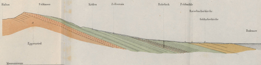
IV. Profil des Bohrloches bei S t Gallen Mafsstab 1 : 500.
