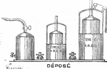
Appareils à produire le gaz hydrocarboné sans mécanique.
