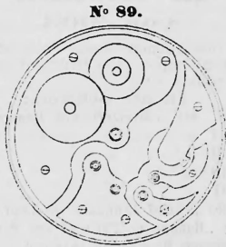
N° 10779. 27 avril 1904, 8 h. p. — Ouvert. — 2 modèles. — Calibres de montres. — Société Anonyme de la Fabrique d'horlogerie Girard-Perregaux & C e , Chaux-de-Fonds (Suisse).
