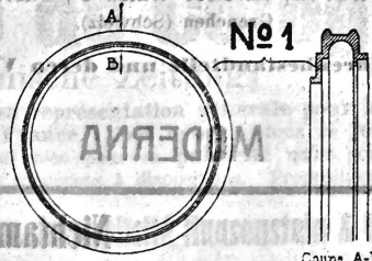
Coupe A-B
