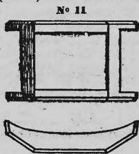
N° 44308. 3 mai 1929, 20 h. — Ouvert. — 1 modèle. — Barette à ressort pour boîtes de montres-bracelets. — Henri Ernest Allemant, Evillard (Suisse).
