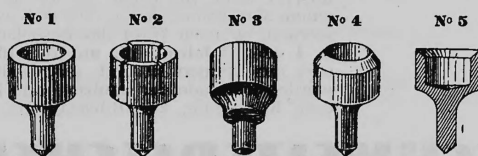
N° 49626. 4 juillet 1932, 11 h. — Ouvert. — 5 modèles. — Tampons creux pour le rhabillage de pivots. — Gustave Beyner, Le Locle (Suisse). Mandataire: Henri Guye, Auvier.
