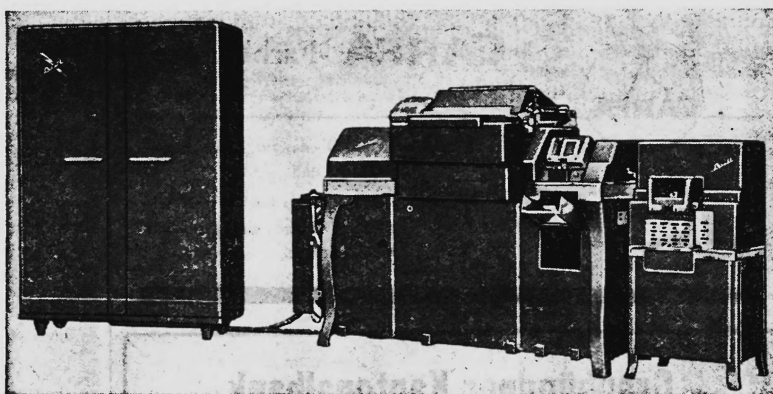
Elektronenrechner GAMMA 3 mit Tabelliermaschine und Blocksummenlocher gekuppelt
