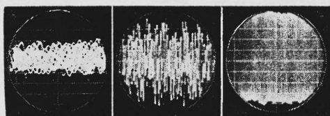
16 kHz 800 kHz 2,3 MHz Kinematische Ultraschallspektren bis 2300 kHz (nach P. Willems)
