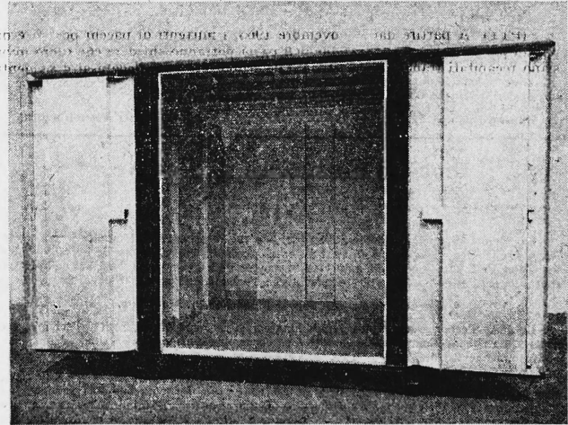
Innenansicht unserer C. T. I. Container Innenmasse: 2,26 x 1,985 x 1,785 m = 8,01 m³
