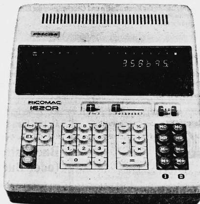
PRECISA-Ricomac 1620 R
