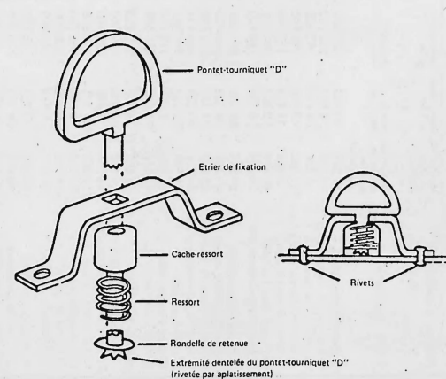
Exemple de pontet-tourniquet (modèle «D»)
