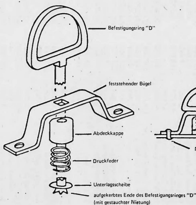
Beispiel eines drehbaren Befestigungsringes (Modell «D»)
